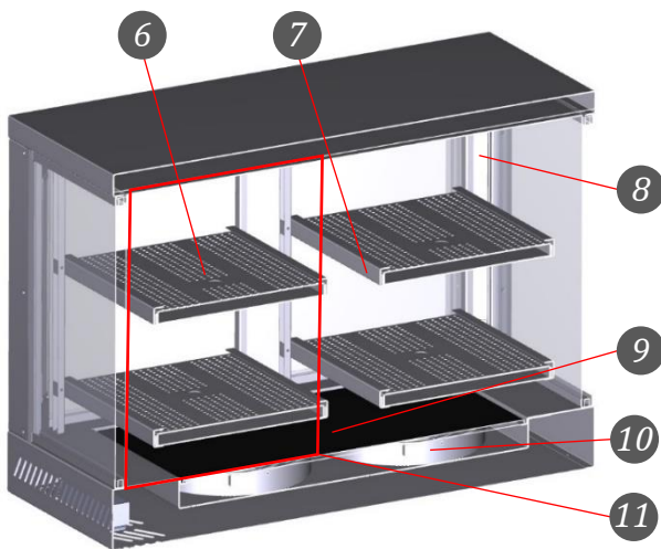
Schnittdarstellung
