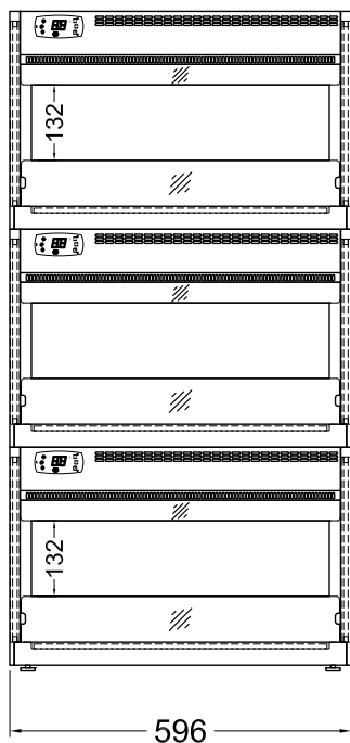
(Voorkant)
