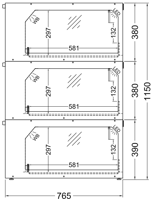
(Zijaanzicht)
