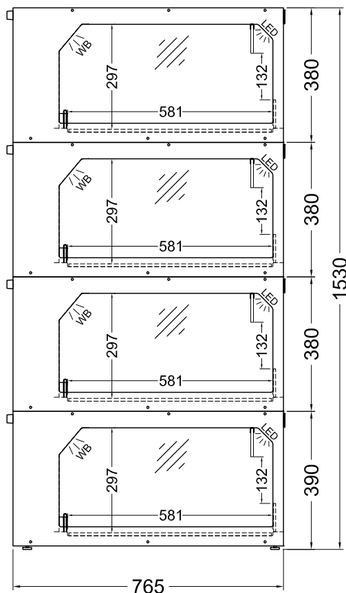
(Zijaanzicht)
