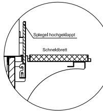
(Detail Spiegelsystem)
