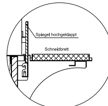
(Detail Spiegelsystem)
