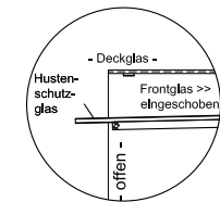
(Detail Spiegelsystem)
