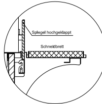
(Detail Spiegelsystem)
